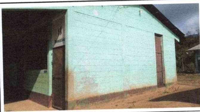
Foto 3: se observa el deterioro de la estructura portante desprendimiento de pintura en las paredes con necesidad de mantenimiento en su totalidad en el modulo 2.
